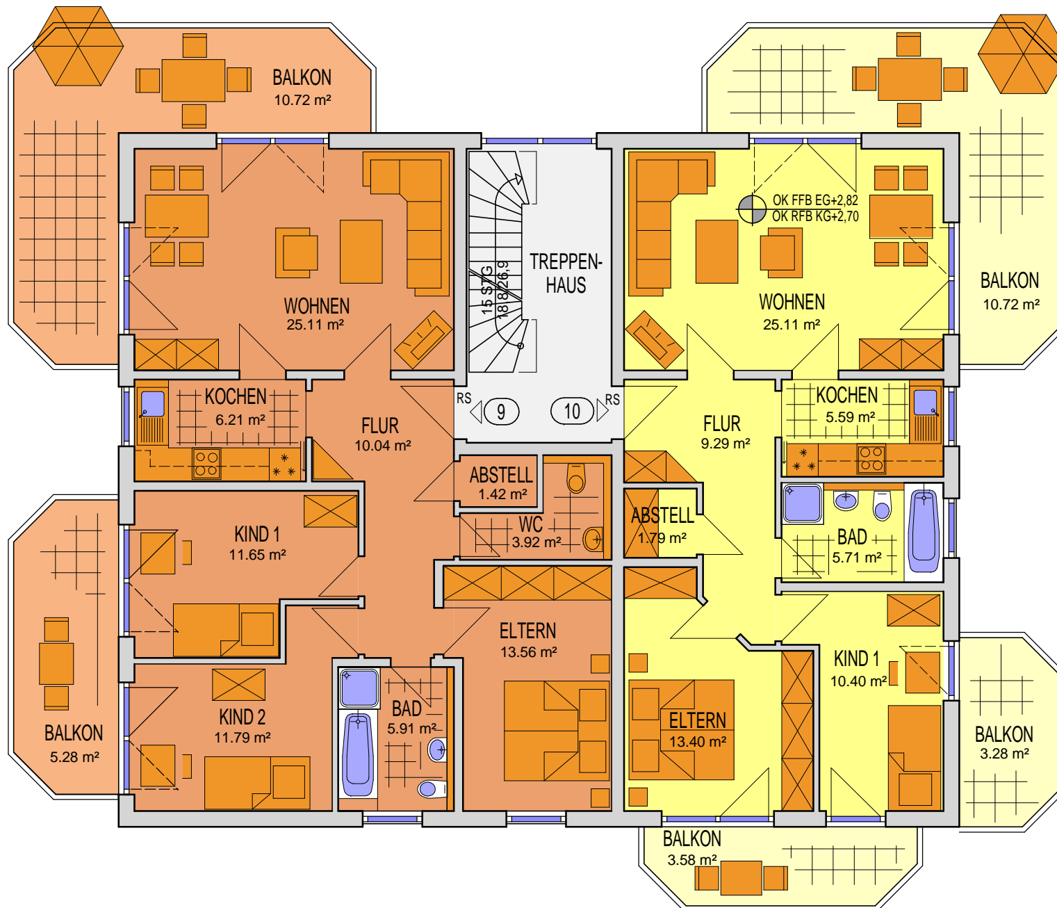
HAUS 2 OG M 1:100
